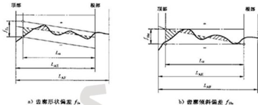
图 2 齿廓偏差
